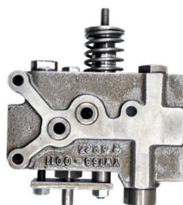
Válvula control levante
