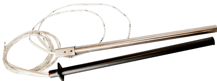
Resistencia para pasteurizador calostros DT60G 3000W square
