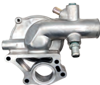
SOPORTE DE LA BOMBA DE AGUA
