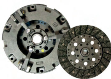
Conjunto de embrague
